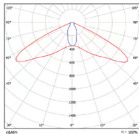
WA-широкая осевая (для BLR 58-58)
