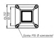
A-A (1 : 5)
