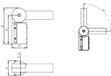
ДКУ кронштейн 02 СБ (вариант монтажа на консоль)
