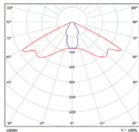
WA-широкая осевая (для BLR 01-58)
