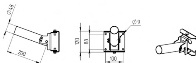
ДКУ кронштейн 03 СБ
