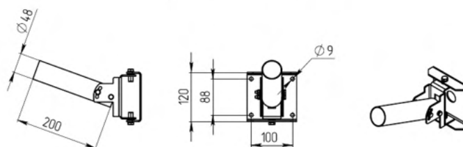
ДКУ кронштейн 03 СБ
